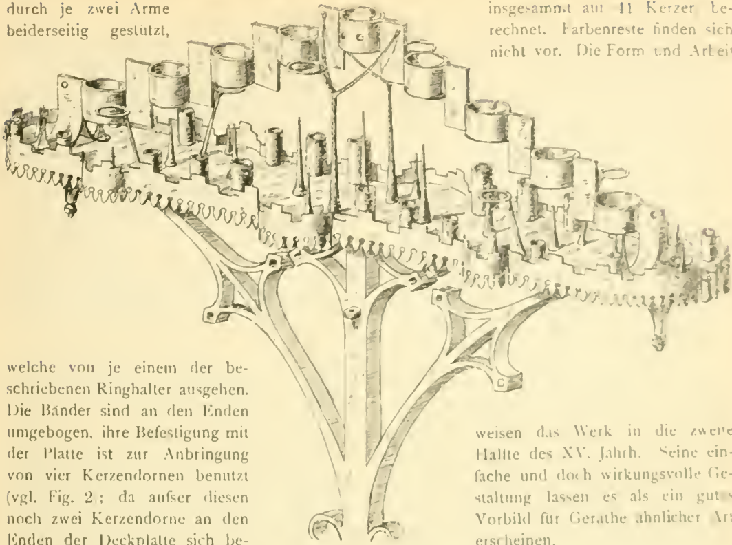
Fig. 2 Perspektivische Theilsicht.
